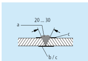
Tompa ragasztás V-varrattal: a=ragasztó b=ragasztószalag közepén védő csíkkal c=poliészter, vagy cellulóz ragasztószalag
